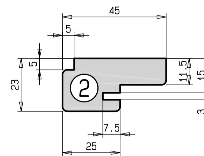
Sonderprofile für Schema G-2 (symmetrisch)
