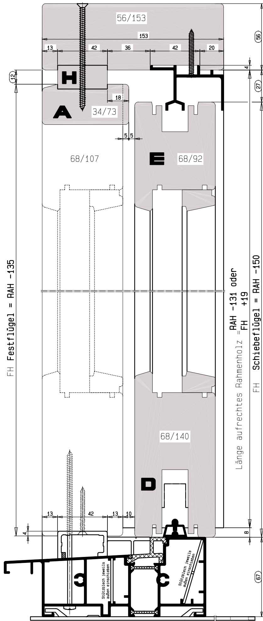
Bodenschwelle HH7642-04 mit Laufschiene HH0131-04
